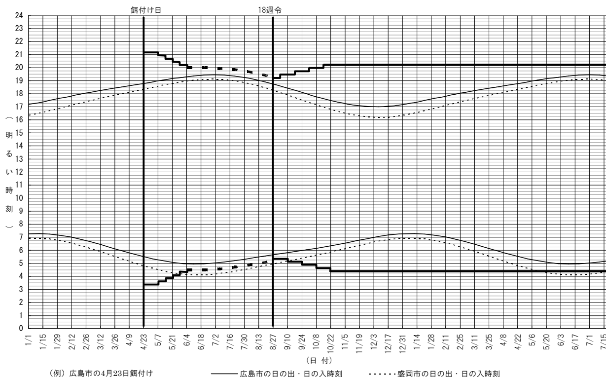
(図4) オープン鶏舎での2月15日から8月18日までにふ化した鶏群の点灯プログラム例
