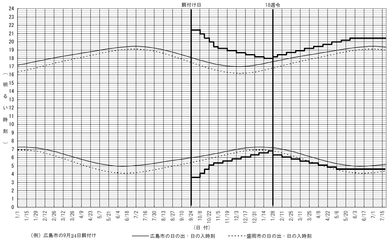
(図5) オープン鶏舎での8月19日から2月14日までにふ化した鶏群の点灯プログラム例
